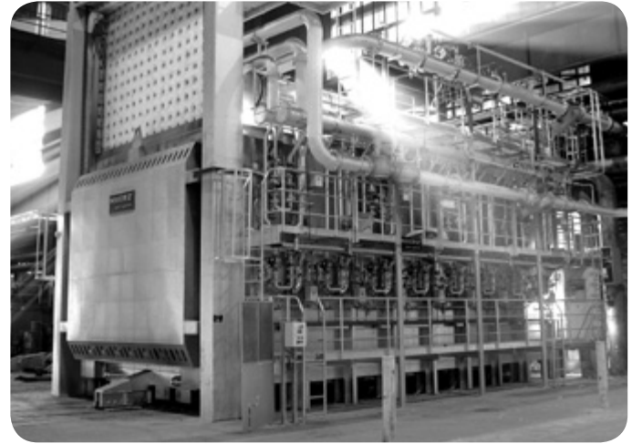
Keramikindustrie: Herdswagenofen
