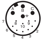
Abb. 1: Servo-Motor: Anschlussbuchse , 14polig (male; Blick auf Servo-Motor)
