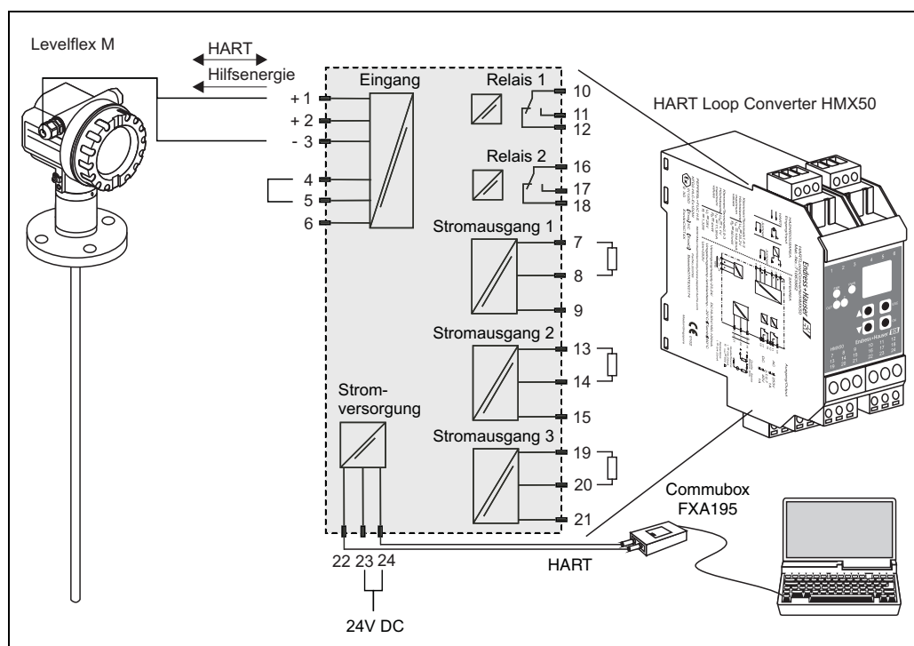
Anschlussschema HART Loop Converter HMX50
