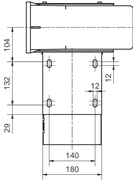
Ansicht A
