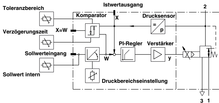
BLOCKSCHALTBIELD (erweitert)
