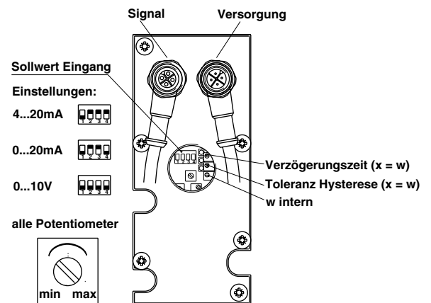
Ausführung mit 2 X Stecker M12
