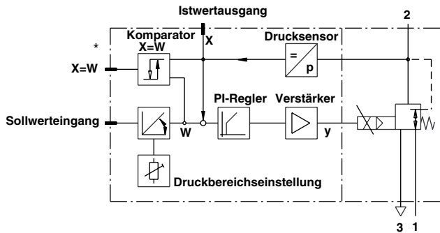
BLOCKSCHALTBILD (Basis)
