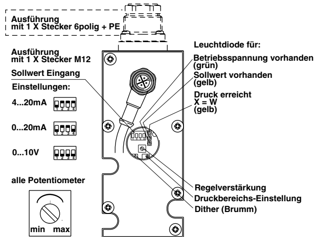
Möglichkeiten der Veränderung der Regelverstärkung bei Anwendungen:
